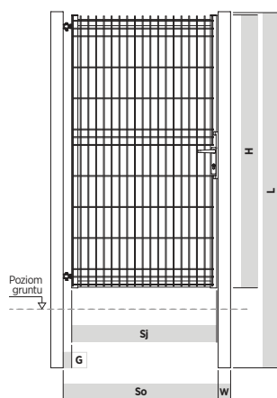
Furтка MODEST widok od wewnątrz
